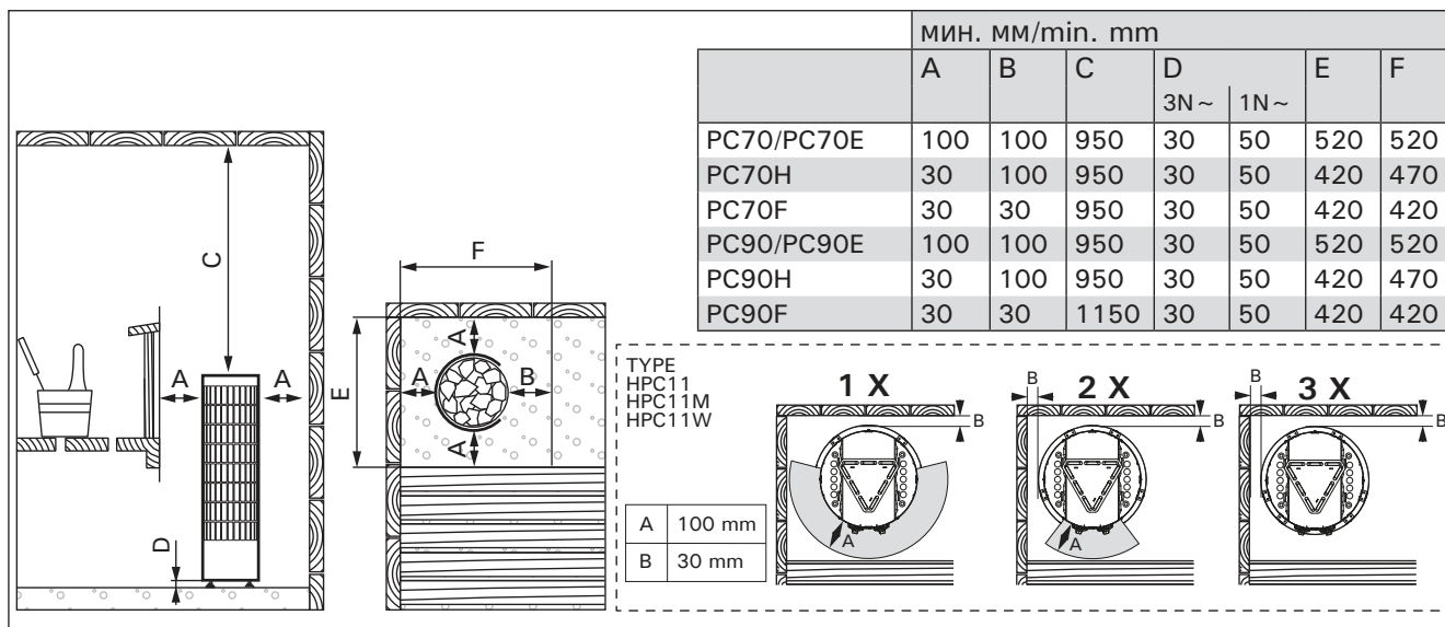
Рисунок 6. Расположение и безопасные расстояния (все размеры приведены в миллиметрах) Joonis 6. Ohutuskaugused (kõik mõõtmised millimeetrites)
