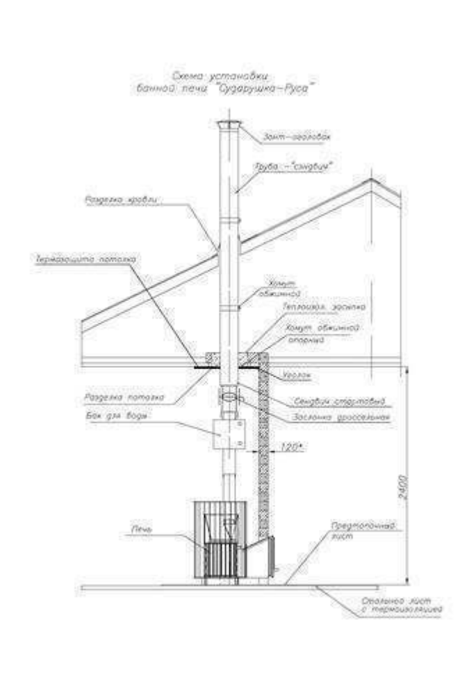
Рис. 4. Схема установки печи
